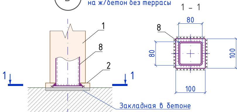
В Установка балясины на ж/бетон без террасы
