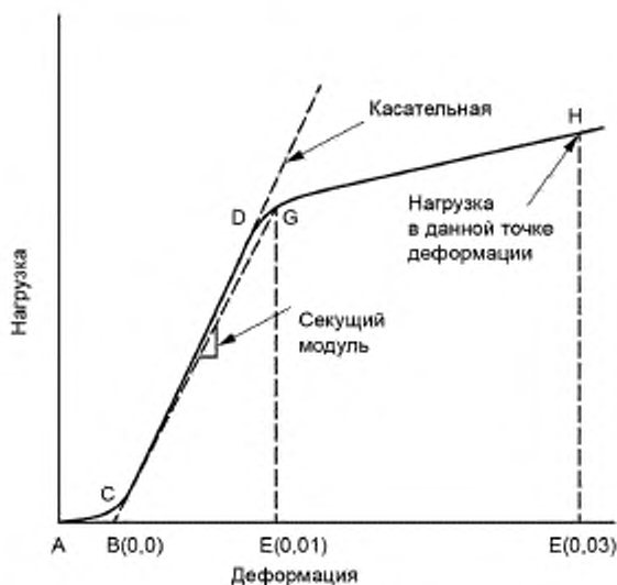
Рисунок Б.1 — График зависимости «нагрузка — деформация»
